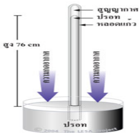
ภาพบารอมิเตอร์
